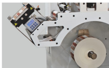
放卷纠偏系统 UNWIND WEB GUIDE
